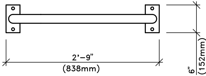
TOP VIEW SCALE: 1"=1'-0"
