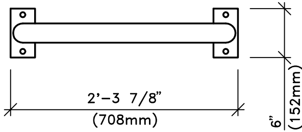
TOP VIEW SCALE: 1"=1'-0"
